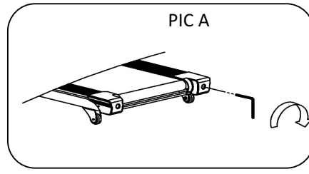
الصورة أ: إذا انحرف الحزام إلى اليمين
